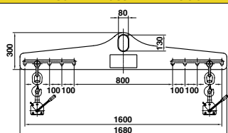
Fixed mini beam MFB 500
